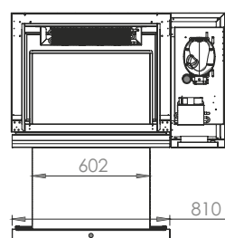
Cooling Counter with Large Drawers Ψυχόμενος Πάγκος με Φαρδιά Συρτάρια
