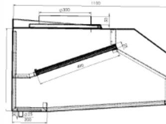
Classic EXTRACTION Hood Κλασική
