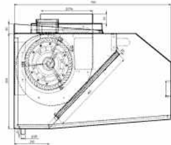
Classic EXTRACTION Hood/with motor Κλασική με ενσωματωμένο μοτέρ
