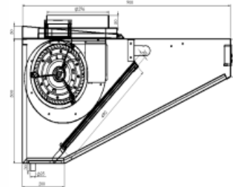
Snack EXTRACTION Hood/with motor Τύπου Snack με ενσωματωμένο μοτέρ
